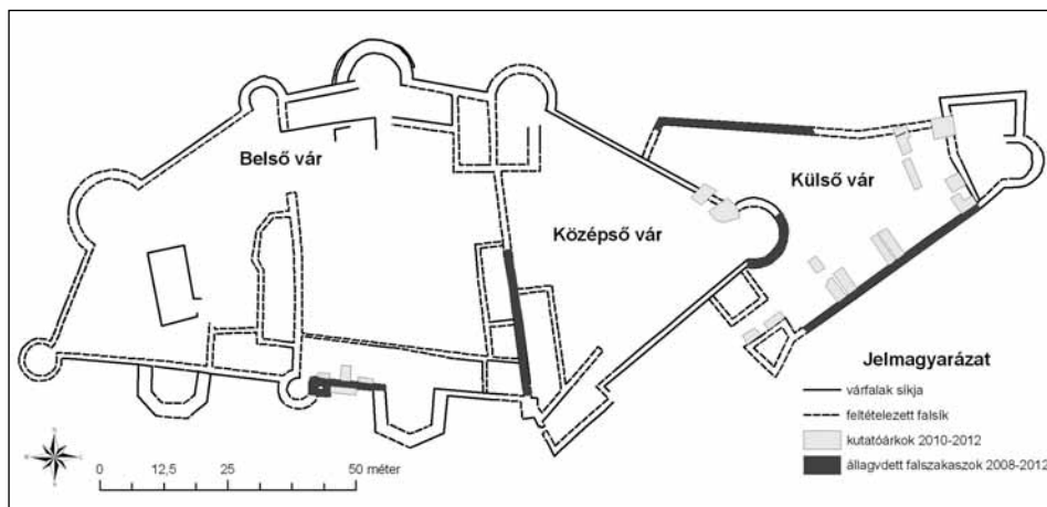
1. kép Szádvár alaprajza a 2008–2012 között végzett állagvédelmi és régészeti munkák jelölésével
